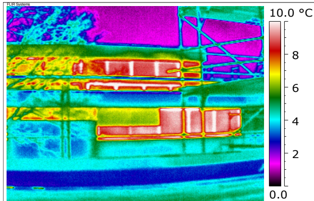
Bauteil: Westfassade, Bauteil B Bemerkungen: Erhebliche Wärmbrücken, undichte Fenster.
