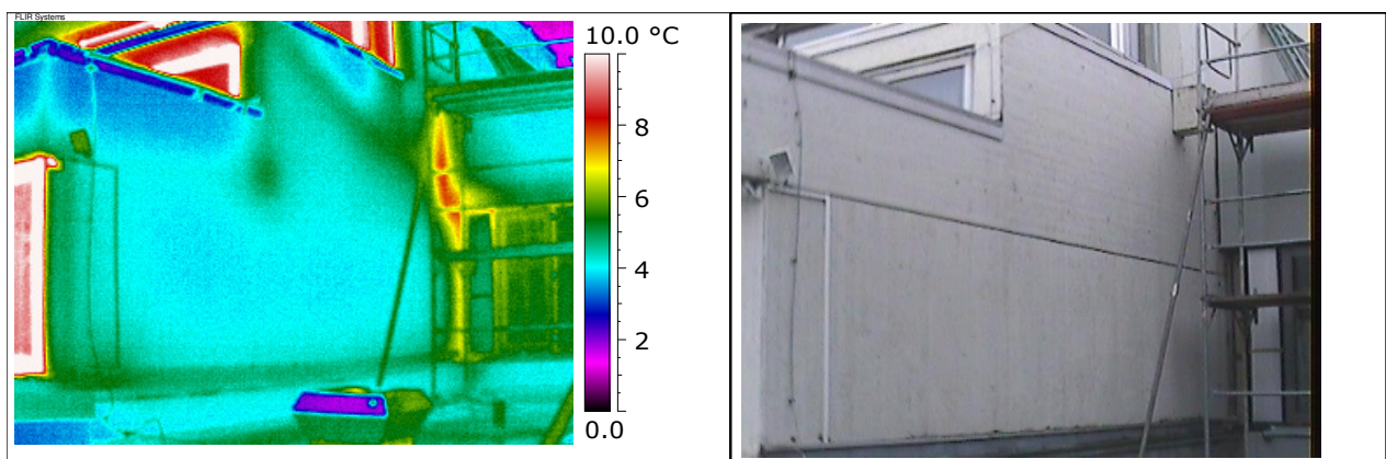
Bauteil: Nordfassade, Bauteil B Bemerkungen: Fassadedämmung unzureichend.
