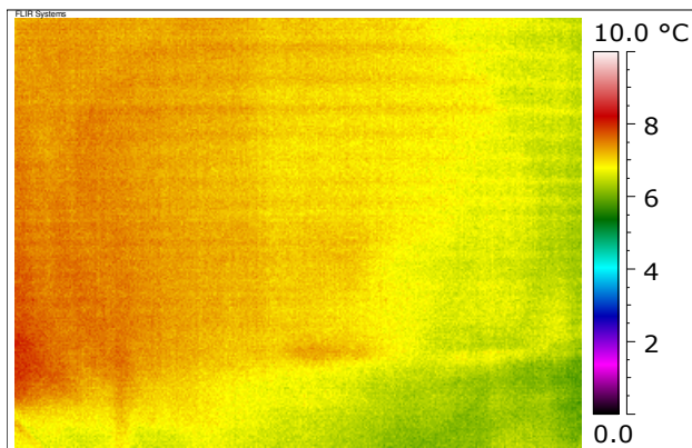
Bauteil: Westfassade, Bauteil B, Passengang Bemerkungen: Erhebliche Wärmbrücken
