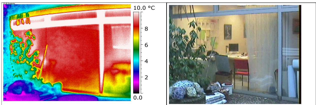
Bauteil: Nordfassade, Verwaltung, Bauteil A Bemerkungen: Undichte Fenster und Türen, Fenster und Türprofile ungedämmt.
