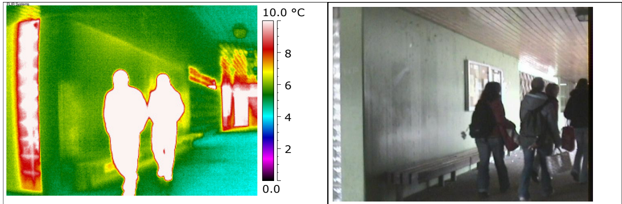
Bauteil: Nordfassade, Verwaltung, Bauteil A Bemerkungen: Fassadedämmung unzureichend.
