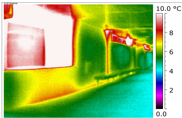
Bauteil: Westfassade, Bauteil B Bemerkungen: Fassadedämmung unzureichend, Erhebliche Wärmbrücken, undichte Fenster.
