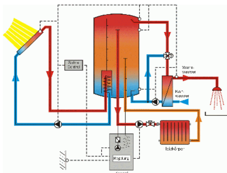
Systemdarstellung der Funktionsweise einer thermischen Solaranlage.
