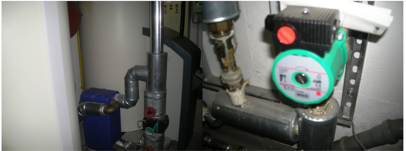
Solar,- und Warmwasserspeicher mit Zirkulationspumpe der Sportanlage
