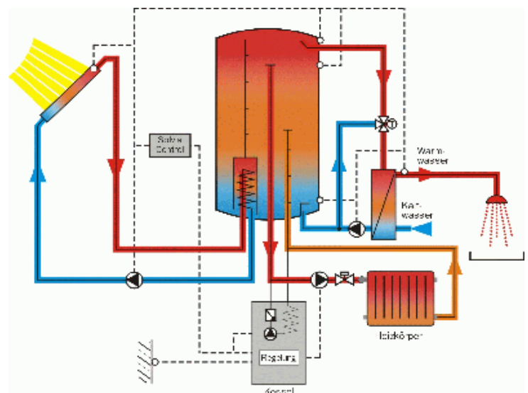
Systemdarstellung der Funktionsweise einer thermischen Solaranlage.
