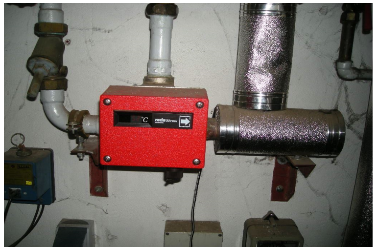
Mischwasserthermostat der Warmwasserbereitstellung
