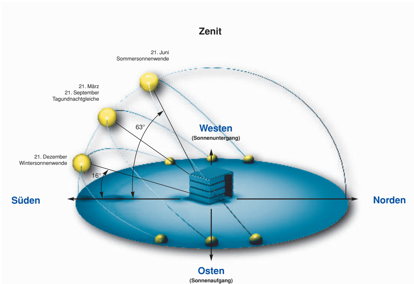
Abb. 1-2: Verlauf der Sonne für Mitteleuropa
